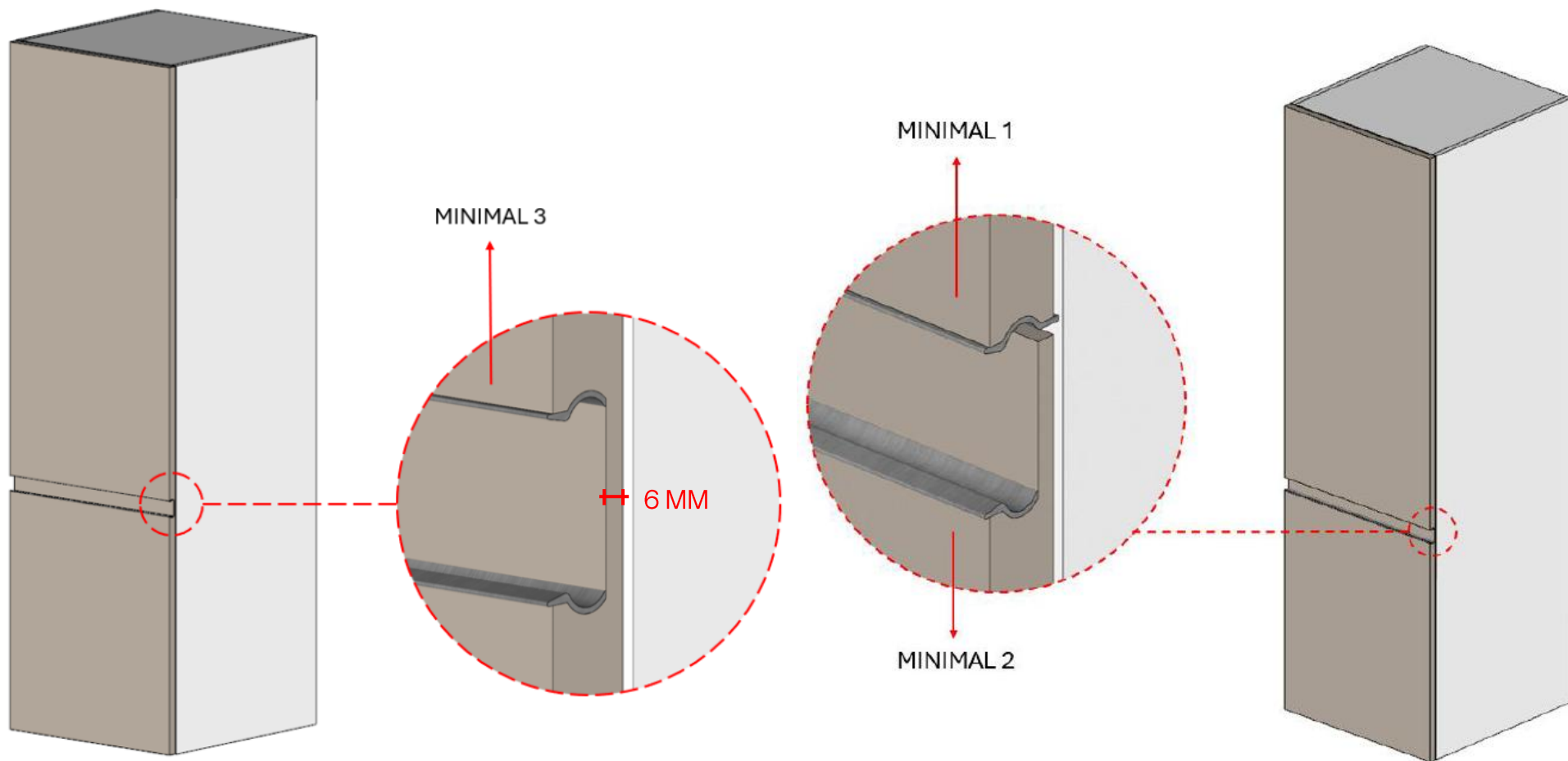
COLUNA PORTA ÚNICA MINIMAL 3 FORA DE LINHA
